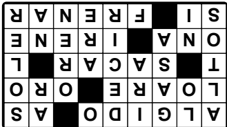
MEZCLAGRAMA
